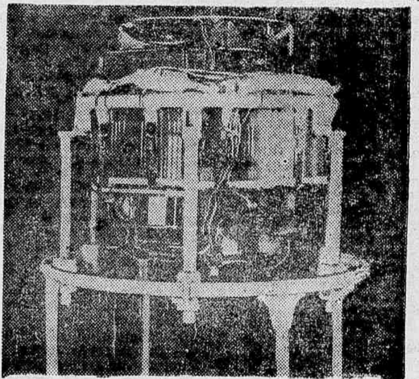
FOGUETE COSMICO — Esta fotografia divulgada há dias em Moscou, reproduz a estrutura do recipiente contido no foguete cósmico, vindo-se as fontes de alimentação dos aparelhos.
