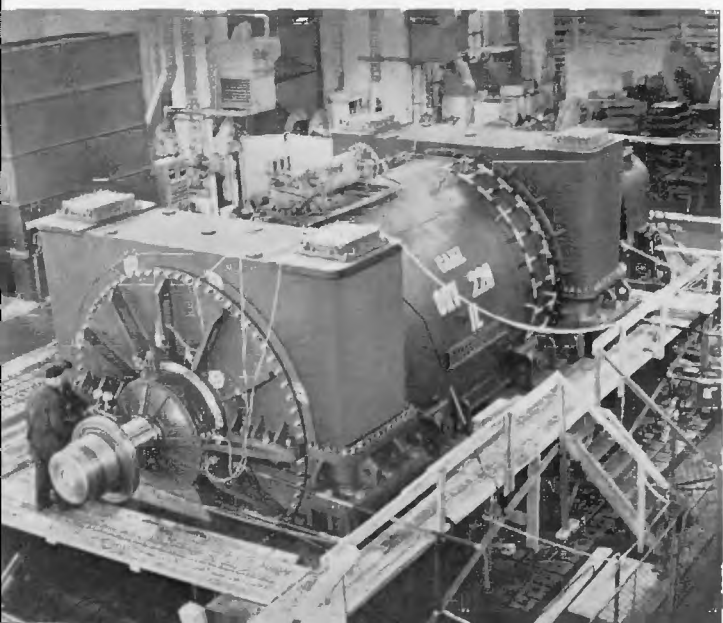
A Ganz Villamossági Művek dolgozói kongresszusi felajánlásként egy hónappal hamarabb elkészítették a Gagarin Hőerőmű 220 megawattos turbógenerátorát
